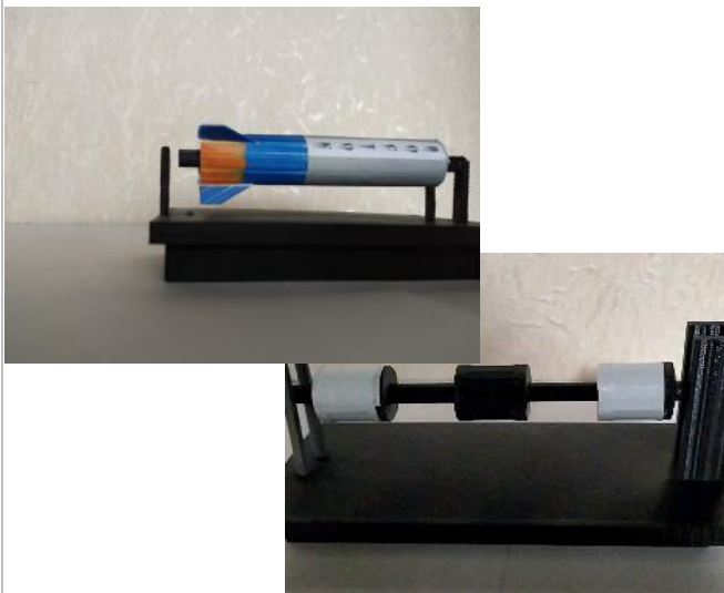
Распечатанный макет «Магнитная подвеска» на 3D принтере Anycubic
