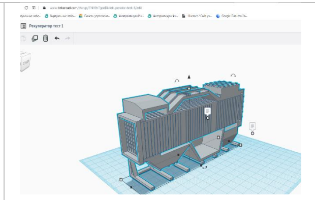
3D рекуператора
